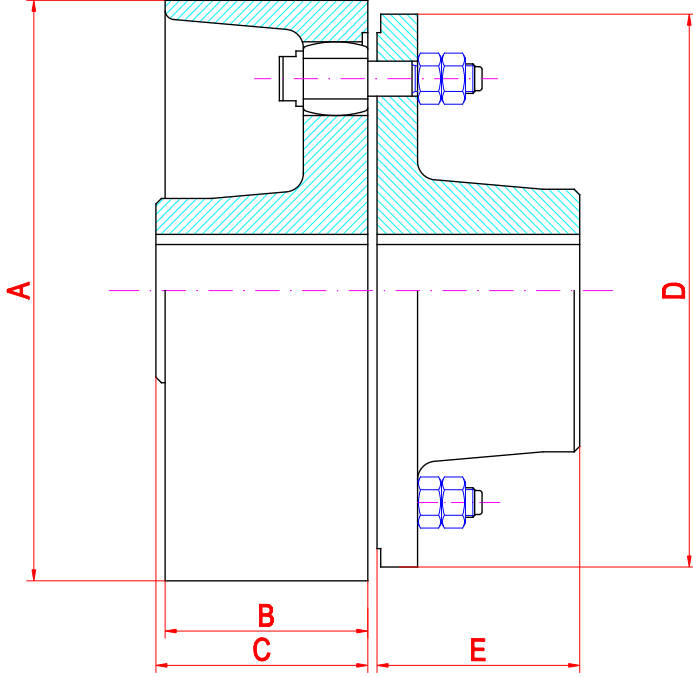
Genel Ölçüler
